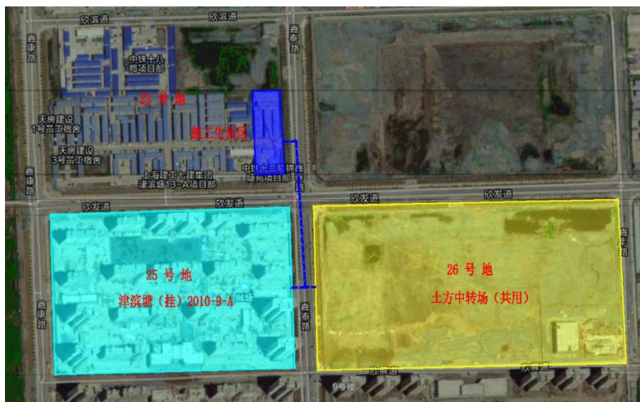
图 1-2 施工生活区及土方中转场位置示意图
