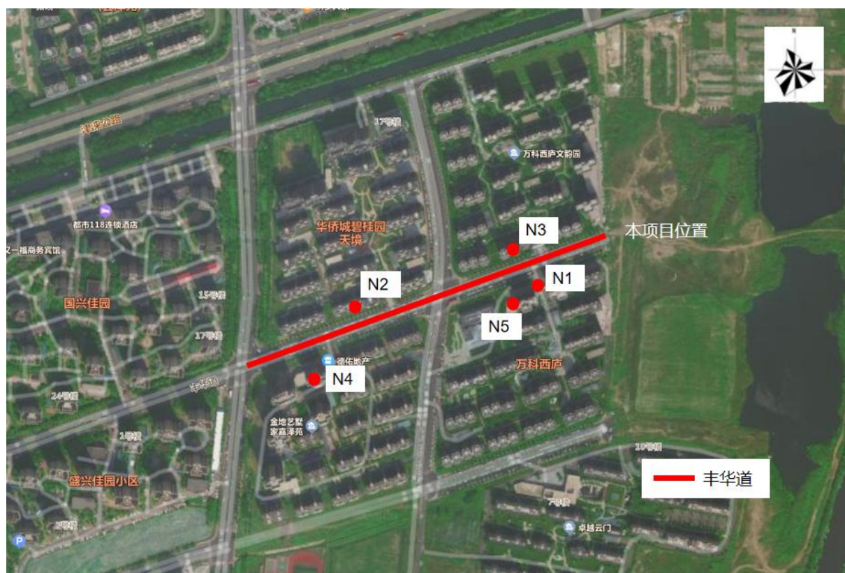
图 6.3-2 丰华道噪声监测点位图
