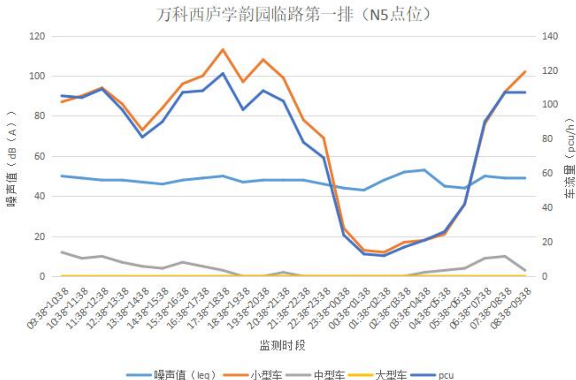
图 6.3-3 24h 监测噪声值和交通量随时间变化的趋势图
